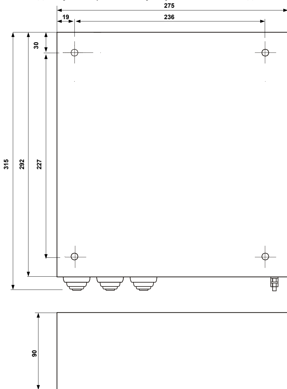
Д Габаритные и установочные размеры изделия «СИГНАЛ-1ДН»
